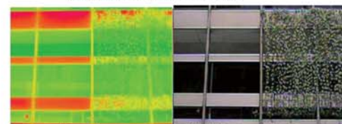
緑のカーテン(遮熱効果の観測)
