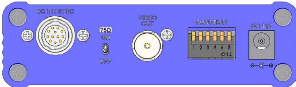
CLA-170 出力側パネル
