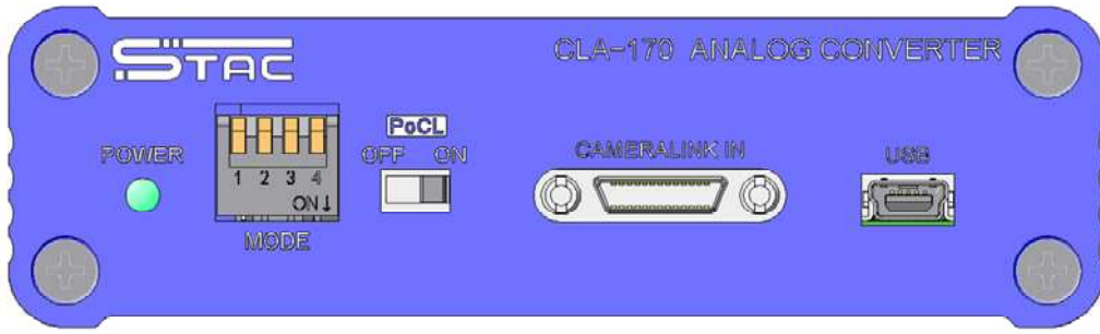
CLA-170 入力側パネル
